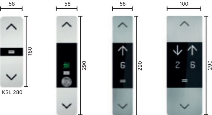
KSL 280 KSL 284 KSL 286 simplex KSL 286 duplex KLX02 Acabamentos: ST4 Silver, aço inoxidável escovado; CB Carbon Black, aço inoxidável escovado (anti-impressão digital)
