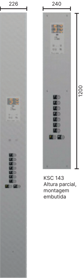
KSC 143 Altura total* montagem embutida
