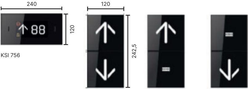
KSH 750 KSI 753 KSA 753 Acabamentos: ST4 Silver, aço inoxidável escovado; CB Carbon Black, aço inoxidável escovado (anti-impressão digital)
